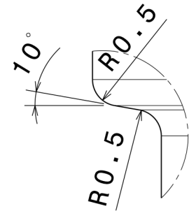
Detail A[2] Scale: 10:1
