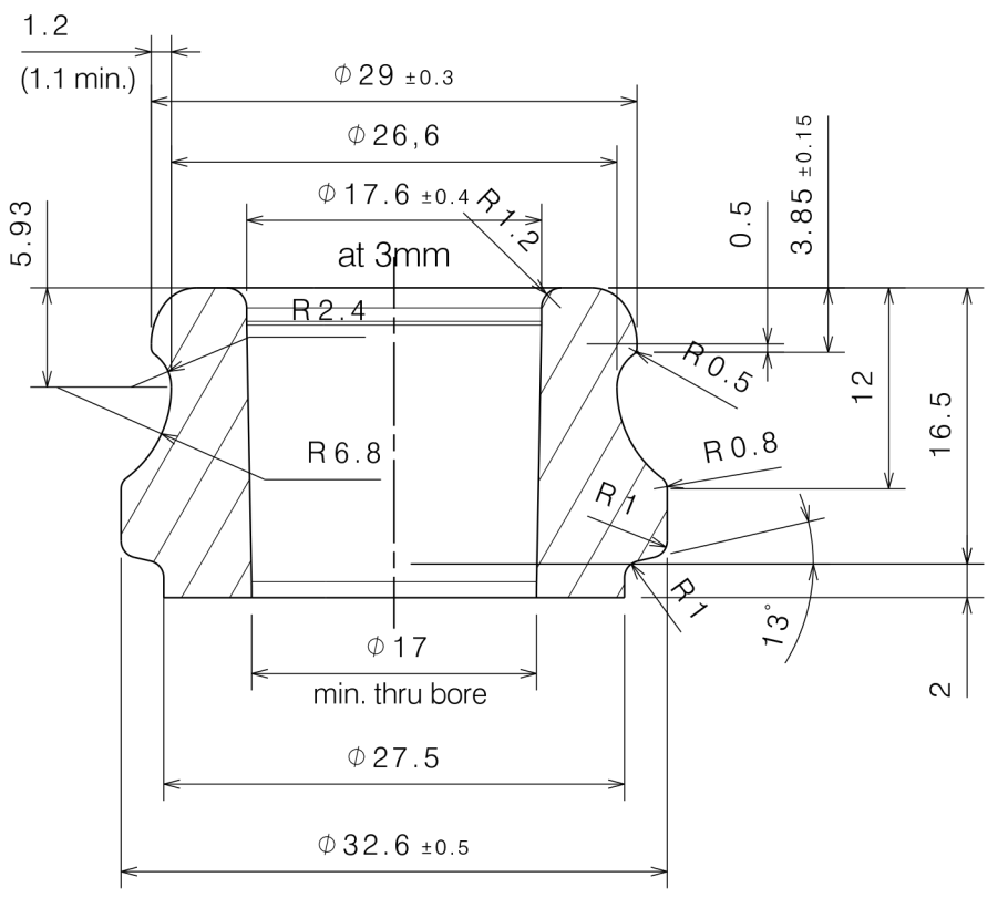
FASCETTA CORONA 26 H 16.5 Scale: 2:1
