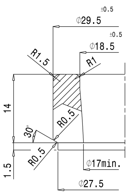
Венчик (2:1) FINISH DETAIL SCALE 2/1
